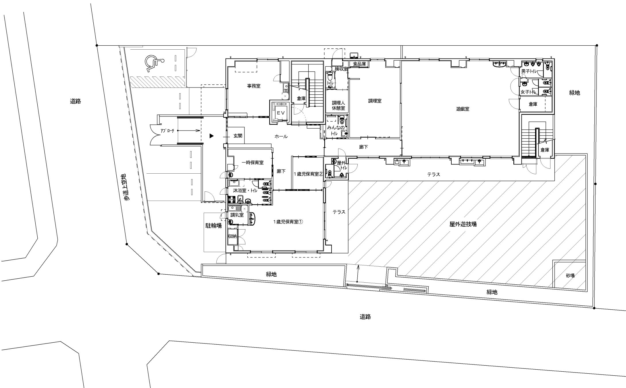
1階 平面図
